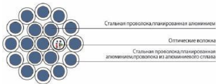
Рисунок 2.11.6.3.2 - Пример оптического кабеля, встроенного в фазный провод
